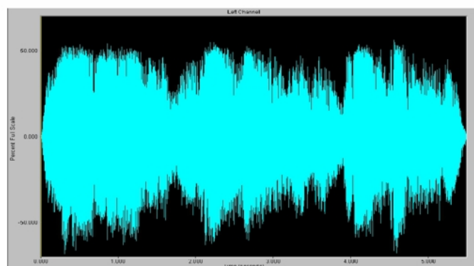
Hallókészülék hangképe telefontekercs ( T ) bemenetről
