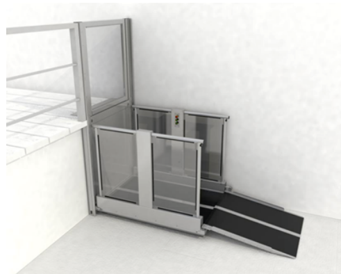
Liftboy 5 elektromos kerekesszék emelő lift
